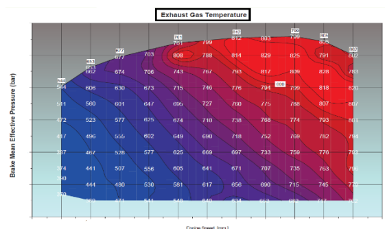
شکل ۱۵) جدول دمای گاز خروجی موتور در دورها و بارهای مختلف بصورت تجربی [۱۷] .
