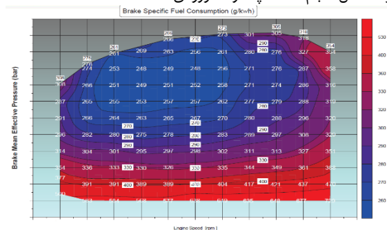
شکل ۱۴) جدول مصرف مخصوص سوخت ترمزی موتور در دورها و بارهای مختلف بصورت تجربی [۱۶] .
