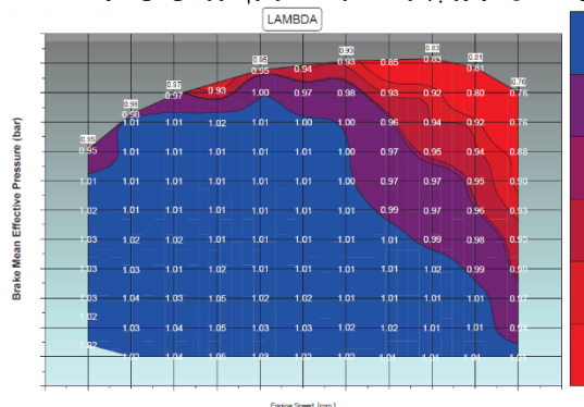
شکل ۲) جدول نسبت هوای اضافی موتور EC5 که در دوره های مختلف محور افقی و بارهای مختلف محور عمودی مقدار نسبت هوای اضافی آمده است.
