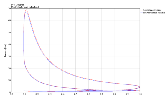
شکل (۱۰) P-V سیلندر یک در دور 6000 rpm و بار کامل در حالت داشتن و نداشتن حجم مشدد چند راهه ورودی
