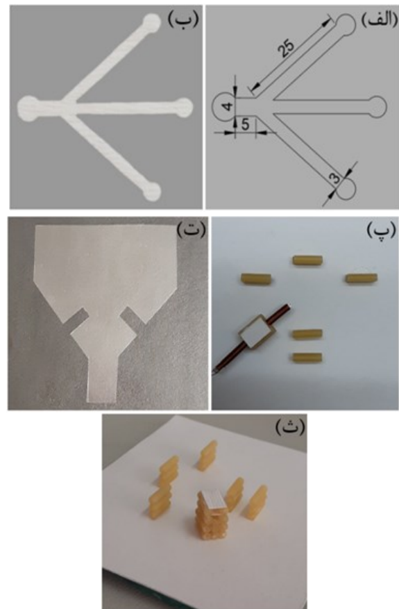
شکل ۳ ساخت ترانزیستور. (الف) طراحی تراشه در نرم‌افزار اتوآکد. (ب) کاغذ برش داده شده با لیزر. (پ) سیم‌پیچ. (ت) ورق پلکسی‌گلاس. (ث) پایه نگاه‌دارنده.
