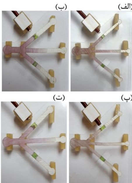
شکل ۷ حجم ۲۰ میکرولیتر برای عبور از محدوده آبریز (۲ و ۳ میلی‌متر) در کانال‌هایی با عرض‌های متفاوت (۲ و ۳ میلی‌متر) کافی نیست (ترانزیستور خاموش). (الف) طول محدوده آبریز ۲ میلی‌متر و عرض کانال ۲ میلی‌متر. (ب) طول محدوده آبریز ۲ میلی‌متر و عرض کانال ۳ میلی‌متر. (پ) طول محدوده آبریز ۳ میلی‌متر و عرض کانال ۲ میلی‌متر. (ت) طول محدوده آبریز ۳ میلی‌متر و عرض کانال ۳ میلی‌متر. کانال بالایی در این شکل دارای ترانزیستور است. در این شکل، کانال بالایی دارای ترانزیستور است. کانال میانی بدون ترانزیستور است. کانال پایینی، کانال آغشته به موم از زیر (بدون سیم‌پیچ) است.
