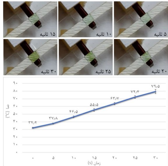
شکل ۵ تاثیر اعمال حرارت توسط سیم‌پیچ بر رفتار موم. ماده سبزرنگ موم است که با اعمال حرارت از زیر کاغذ به داخل آن نفوذ کرده و به سطح تراشه می‌رسد تا کانال را مسدود کند.
