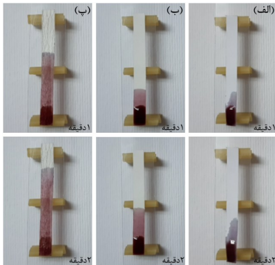
شکل ۲ حرکت سیال در کاغذهای مختلف. (الف) کاغذ A4، (ب) کاغذ فیلتر صاف و (پ) کاغذ فیلتر چروکیده.
