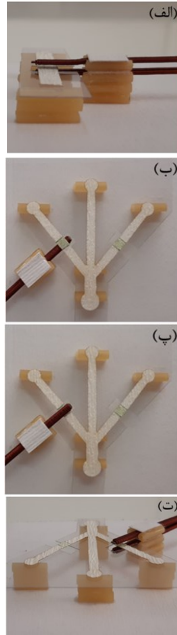
شکل ۳ (الف) شمای جانبی ترانزیستور. (ب) شمای تراشه شامل ترانزیستور (کانال سمت چپ)، کانال کاغذی (کانال میانی) و کانال کاغذی آغشته به موم (کانال سمت راست). در این شکل سیم‌پیچ بالایی به منظور نمایش سیم‌پیچ پایینی حذف شده است. (پ) شمای تراشه شامل ترانزیستور (کانال سمت چپ)، کانال کاغذی (کانال میانی) و کانال کاغذی آغشته به موم (کانال سمت راست). در این شکل ترانزیستور کامل نمایش داده شده است. (ت) نمای جانبی تراشه نمایش داده شده است.
