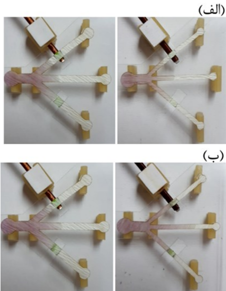
شکل ۶ ترانزیستور در حالت خاموش (الف) حجم ۱۰ میکرولیتر برای تراشه‌ای با عرض ۲ و ۳ میلی‌متر، (ب) حجم ۱۵ میکرولیتر برای تراشه‌ای با عرض ۲ و ۳ میلی‌متر. در این شکل، کانال بالایی دارای ترانزیستور است. کانال میانی بدون ترانزیستور است. کانال پایینی، کانال آغشته به موم از زیر (بدون سیم‌پیچ) است.
