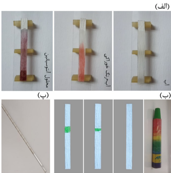
شکل ۴ (الف) استفاده از سیالات مختلف بر روی کاغذ. (ب) استفاده از مدادشمعی به عنوان ماده آبگریز. (پ) پیپت به منظور انتقال حجم مناسب سیال بر روی تراشه.
