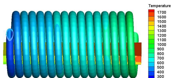
شکل ۱۵) کانتور دما روی لوله‌های مارپیچ و سرباره
