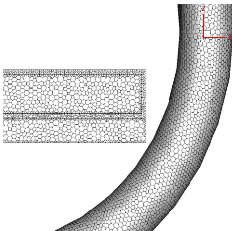
شکل ۱۰) نمایی نزدیک از شبکه‌ی محاسباتی
