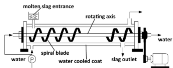
شکل ۳) روش همزن مکانیکی توسعه یافته [3]
