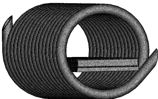
شکل ۹) نمایی از شبکه‌ی محاسباتی ایجاد شده روی لوله‌های مارپیچ، سرباره و نوار نقاله
