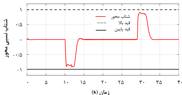
شکل ۵) حفظ قید مربوط به شتاب موتور
