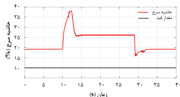
شکل ۷) حفظ قید مربوط به حاشیه سرج کمپرسور
