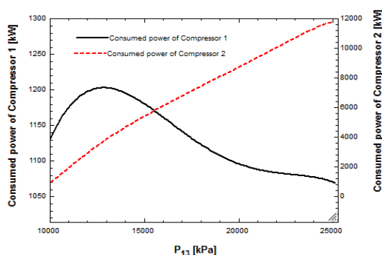
شکل ۲) تاثیر تغییرات فشار ورودی به توربین بر عملکرد ترمودینامیکی کلی سیکل ترکیبی تولید توان و تبرید تراکمی دارای اجکتور با سیال عامل دی اکسید کربن
