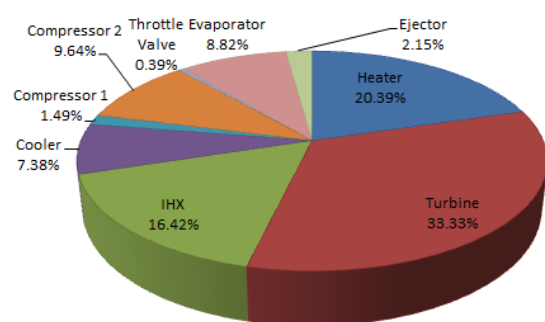
شکل ۶) سهم اجزای مختلف سیکل ترکیبی تولید توان و تبرید تراکمی دارای اجکتور با سیال عامل دی اکسید کربن در نرخ تخریب اگزرژی کل
