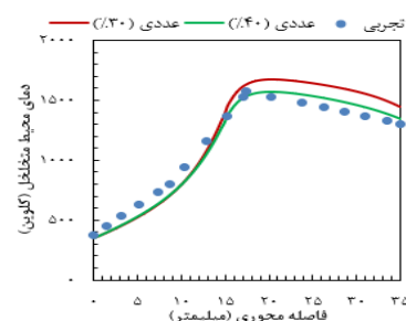
شکل ۴) نمودار دمای عددی و تجربی در فاصله ۲۰ میلیمتری دیوار مشعل
