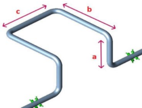
شکل ۳) شکل و ابعاد حلقه انبساط
