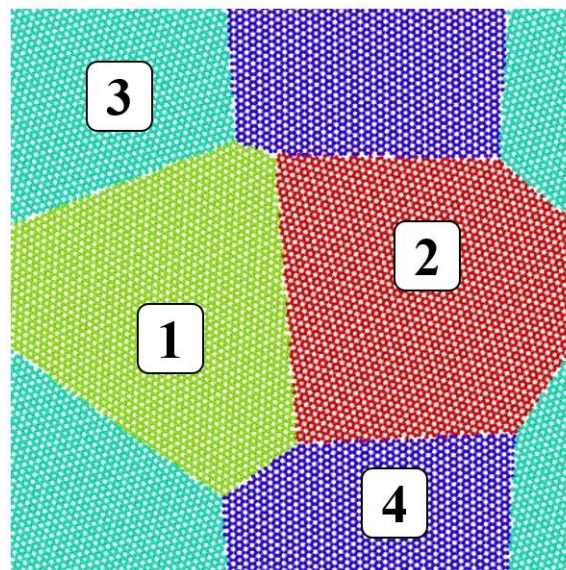
شکل ۲ ساختار پلی کریستال نیتريد بور با ۴ ناحیه در حضور مرزدانه ها
