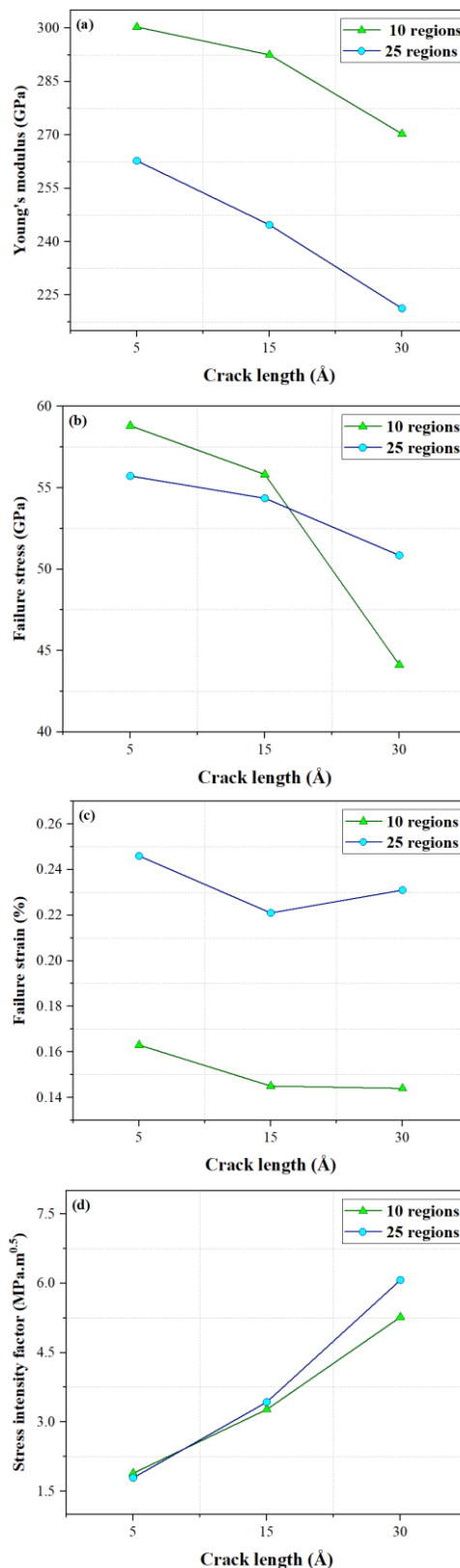
شکل ۸ الف) مدول یانگ، ب) تنش شکست، ج) کرنش شکست، د) شدت تنش پلی کریستال نیتريد بور با ۱۰ و ۲۵ ناحیه، تحت تاثیر طول‌های ترک مختلف
