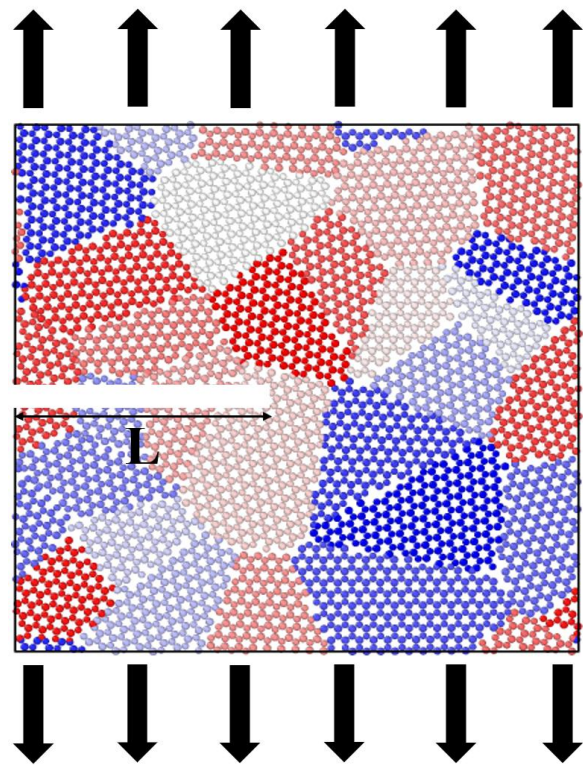
شکل ۷ محل قرارگیری ترک با طول L و جهت بارگذاری در راستای Y Fig. 7 The location of edge crack and loading along Y direction
