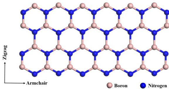
شکل ۱ نمای بالا از ساختار نیتريد بور که در آن، راستای کشش در جهت X و Y به ترتیب آرمچير و زيگزاگ معرفی شده است.
