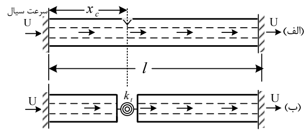
شکل ۴ (الف) لوله ترک‌دار حامل سیال، (ب) مدل ریاضی لوله ترک‌دار حامل سیال
