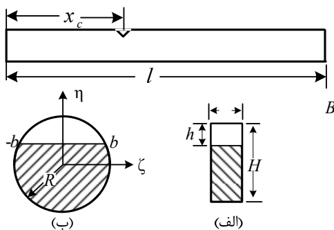
شکل ۱ تیر ترک‌دار با (الف) سطح مقطع مستطیلی، (ب) سطح مقطع دایره‌ای
