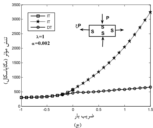
شکل ۵ منحنی ضریب بار ( \xi ) بر حسب تنش مؤثر ( \sigma_e )
