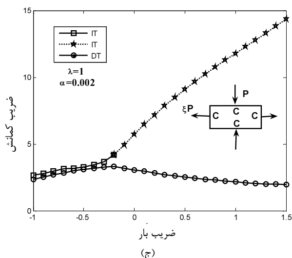
شکل ۱۲ مقایسه تئوریهای نموی و تغییرشکل برای حالت CCCC
