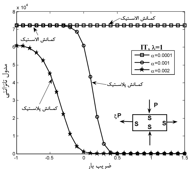
شکل ۷ منحنی مدول تانژانتی - ضریب بار تئوری نموی
