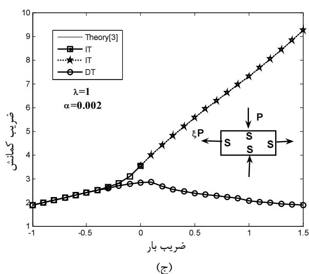
شکل ۴ مقایسه تئوریهای نموی و تغییر شکل برای حالت SSSS
