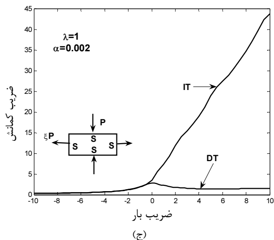
شکل ۶ اثر ضریب بار بر ضریب کمانش براساس دو تئوری نموی و تغییر شکل
