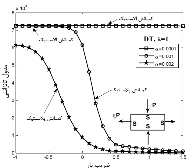
شکل ۸ منحنی مدول تانژانتی - ضریب بار تئوری تغییر شکل
