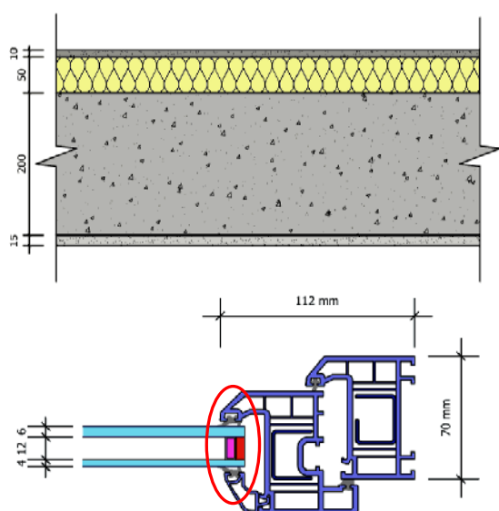
شکل ۱ دیوار نمونه و مقطع افقی پنجره جهت انجام محاسبات
