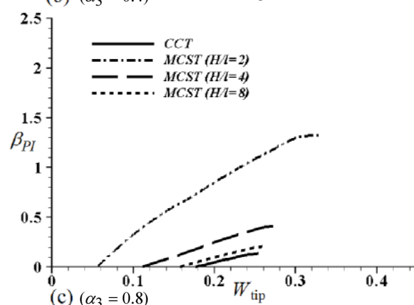
شکل ۸ تغییرات خیز انتهایی تیر بر اساس ولتاژ پولین به همراه اثر اندازه برای مقادیر مختلف نیروی واندروالس
