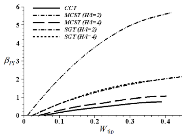
شکل ۱۰ تغییرات خیز انتهایی تیر بر اساس ولتاژ پولین به همراه اثر اندازه برای نیروی واندروالس \alpha_3 = 0.4
