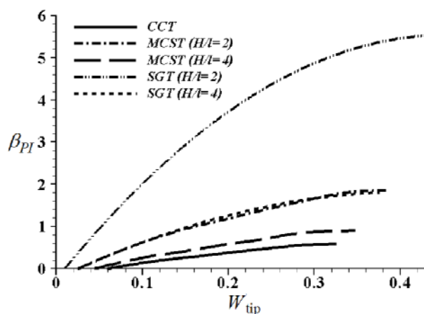
شکل ۹ تغییرات خیز انتهایی تیر بر اساس ولتاژ پولین به همراه اثر اندازه برای نیروی کازمیر \alpha_4 = 0.4
