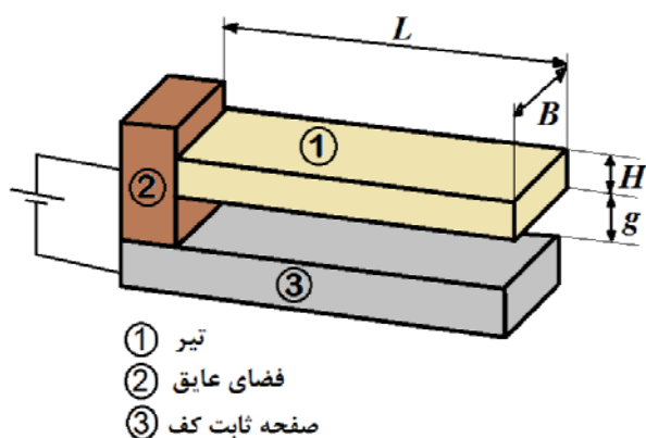
شکل ۱ طرحواره نانوعملگر
