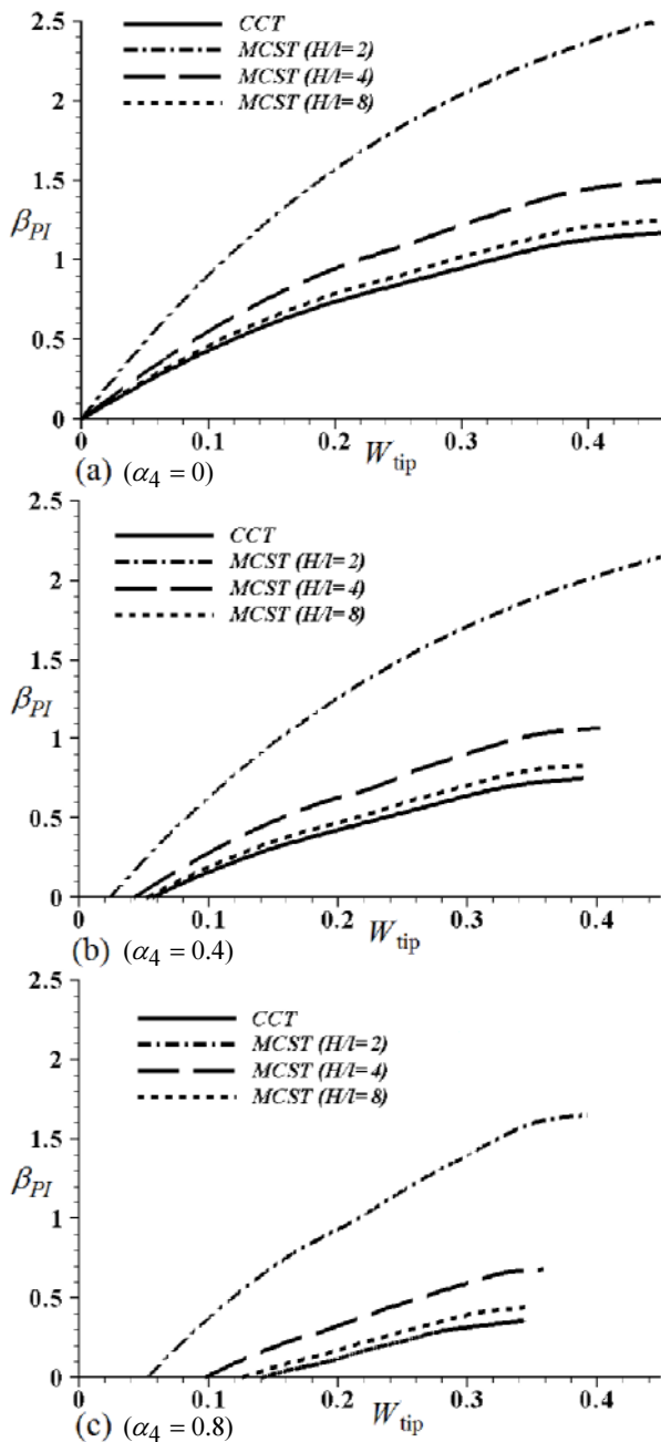
شکل ۷ تغییرات خیز انتهای تیر بر اساس ولتاژ پولین به همراه اثر اندازه برای مقادیر مختلف نیروی کازمیر
