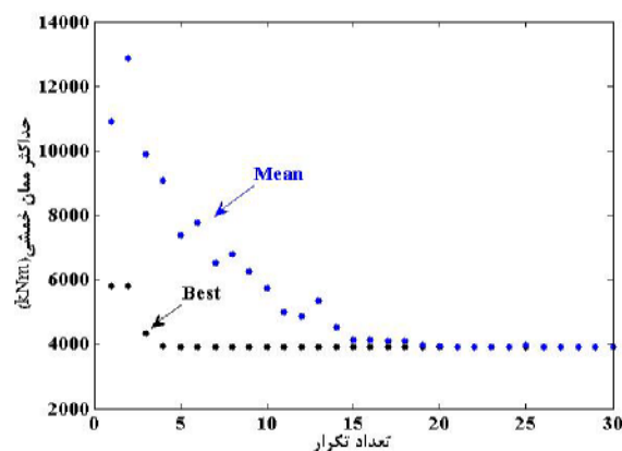
شکل ۸ روند رسیدن به سازه بهینه برای سازه اسکلتی حالت دوم
