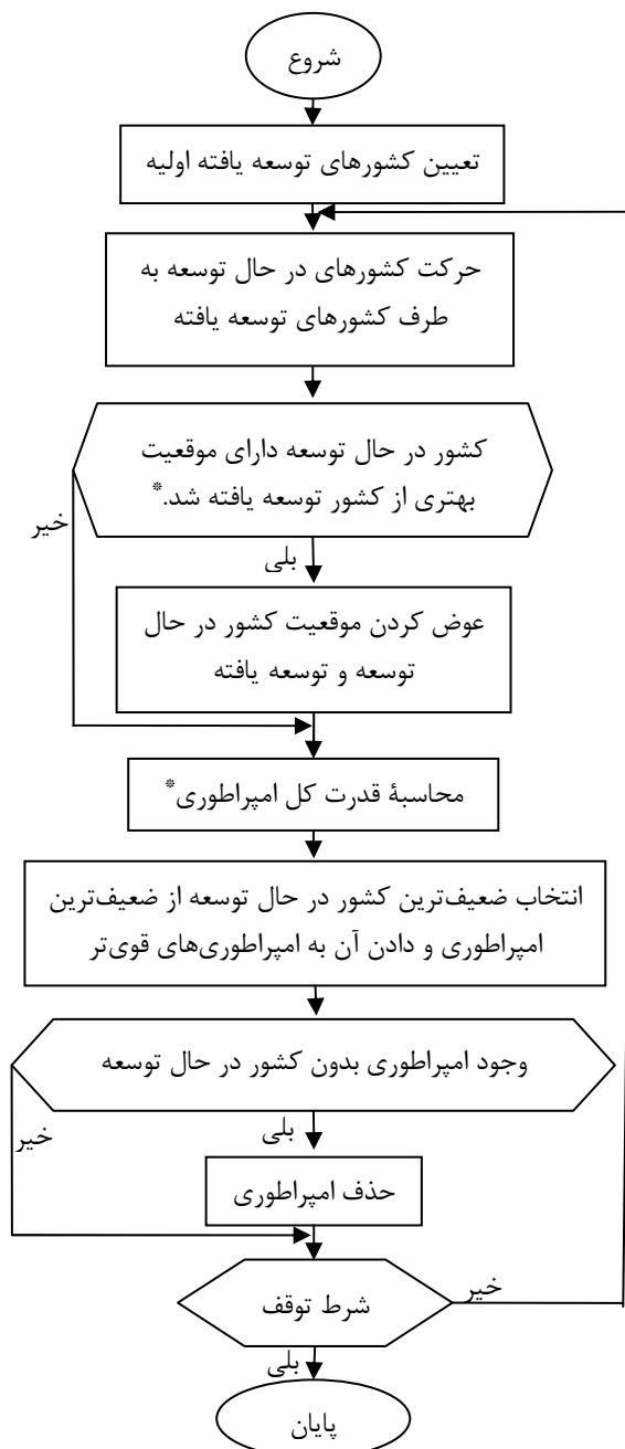
شکل ۲ فلوچارت روش بهینه‌سازی رقابت استعماری
