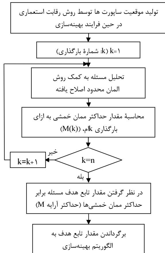
شکل ۳ فلوچارت چگونگی محاسبه تابع هدف در مسئله
