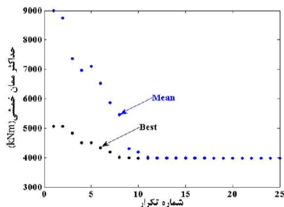
شکل ۷ روند رسیدن به سازه بهینه برای سازه اسکلتی حالت اول
