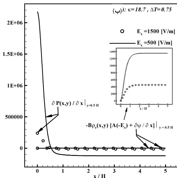
شکل ۵ گرادیان فشار و نیروی الکتریکی لورنس
