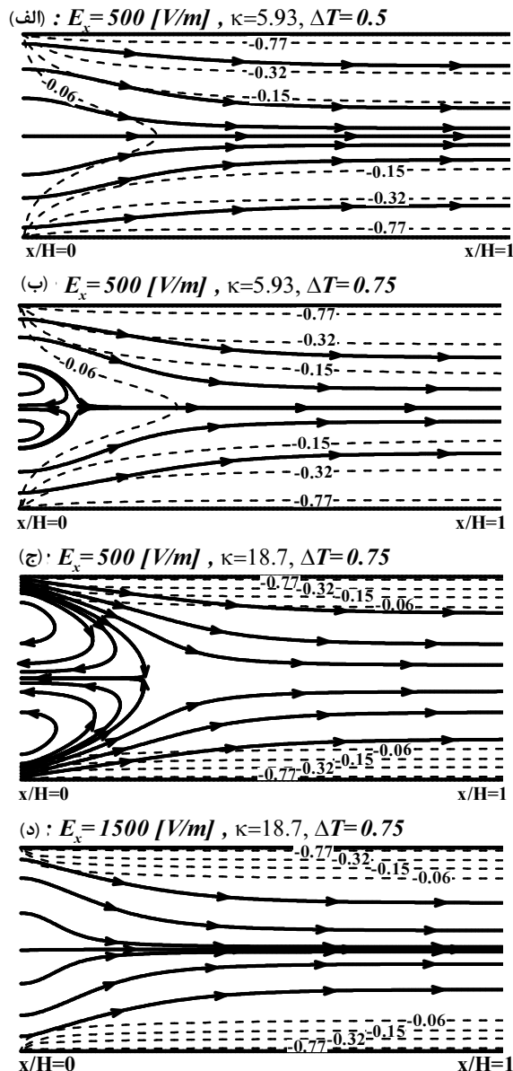
شکل ۴ طرح جریان الکترواسمتیک و پتانسیل الکتریکی داخلی، خطوط ممتد خطوط جریان الکترواسمتیک و خطچین خطوط پتانسیل الکتریکی داخلی ثابت
