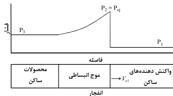
شکل ۲ پروفیل فشار در یک لحظه از زمان در طول استوانه [۹]
