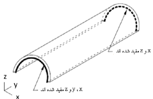
شکل ۴ شرایط مرزی مدنظر برای استوانه جدار نازک
