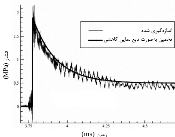
شکل ۱ پروفیل واقعی موج دتونییشن (اندازه گیری شده در آزمایشگاه) و معادل ایده آل آن [۱]
