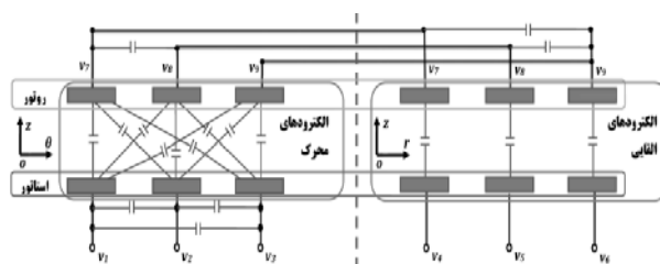
شکل ۴ مدل در نظر گرفته شده برای تحلیل محرک
