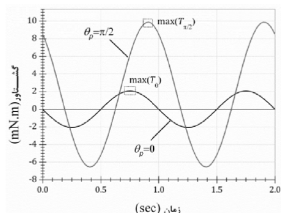
شکل ۷ نمودار تغییرات گشتاور برای مکان ثابت \theta_p = 0, \frac{\pi}{2}
