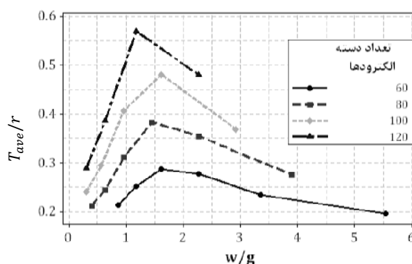
شکل ۹ تغییر نسبت \frac{T_{ave}}{r} بر حسب متغیرهای طراحی
