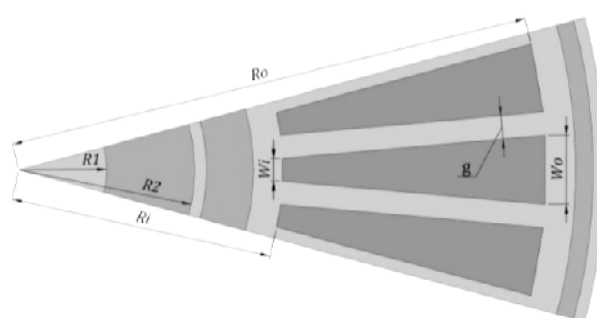
شکل ۵ پارامترهای طراحی الکترودها در قطاعی از بردها که نشان دهنده یک دسته الکترودها است.
