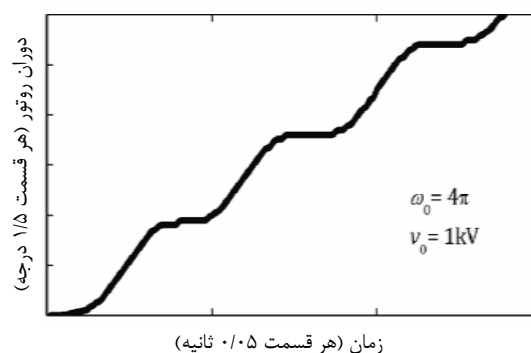
شکل ۱۵ نحوه حرکت واقعی موتور
