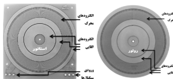
شکل ۱۱ بردهای ساخته شده برای روتور و استاتور
