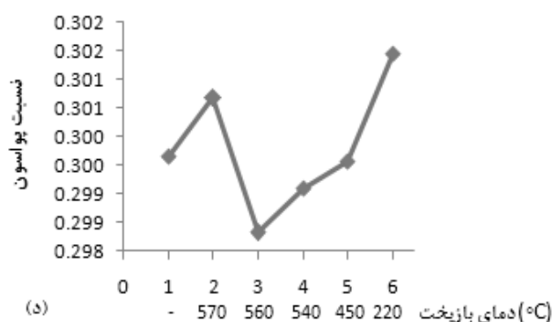
شکل ۷ تاثیر دمای بازپخت بر روی خواص مکانیکی نمونه‌های فولاد AISI D6: (الف) مدول برشی (ب) مدول ینگ (ج) مدول حجمی (د) نسبت پواسون
