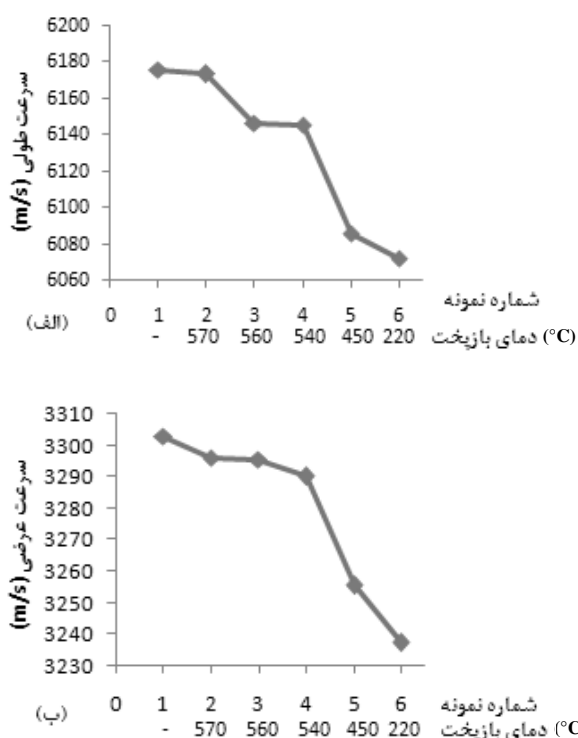
شکل ۶ خواص فراصوتی نمونه‌های فولاد AISI D6، (الف) سرعت طولی (ب) سرعت عرضی
