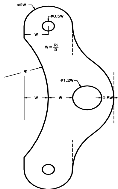
شکل ۴ هندسه نمونه پیشنهادی جدید بر اساس ملاحظات مکانیک شکست
