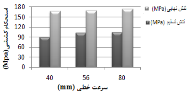
شکل ۹ تاثیر سرعت خطی ابزار بر مقدار استحکام کششی
