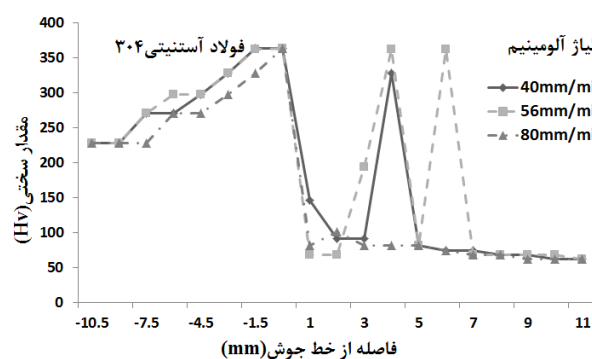
شکل ۷ تاثیر سرعت‌های خطی مختلف در مقدار سختی
