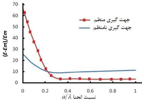
شکل ۹ میزان تغییر مدول موثر با نسبت انحنای برای درصد حجمی ۰/۳ و نسبت طول به قطر ۳۰۰
