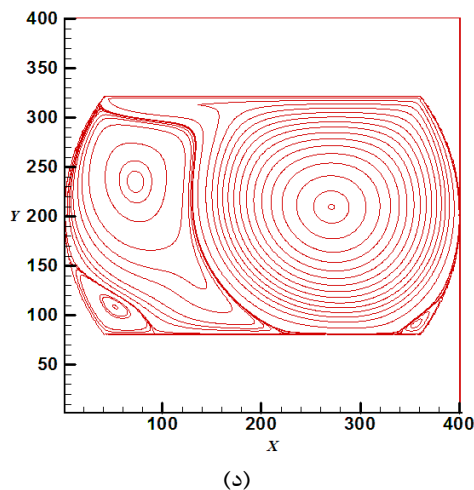
شکل ۹ (الف) خطوط جریان در Re=400 ، (ب) خطوط جریان در Re=1000 ، (ج) خطوط جریان در Re=2000 ، (د) خطوط جریان در Re=4000
