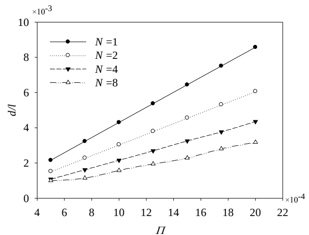
شکل ۴ ضخامت رویه ( d/l ) برحسب شاخص بار H/l برای تعداد آرایه‌های مختلف ( N )
