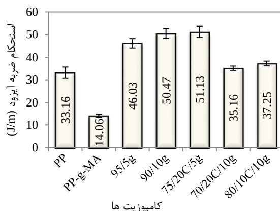
شکل ۹ استحکام ضربه آیزود حالت‌های خالص و ترکیب‌های دوتایی و سه‌تایی پلی‌پروپیلن، PP-g-MA و \text{CaCO}_3
