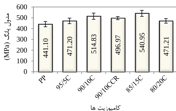
شکل ۸ مدول یانگ ترکیب‌های دوتایی پلی پروپیلن و نانوذرات کربنات کلسیم در درصد‌های وزنی مختلف کربنات کلسیم
