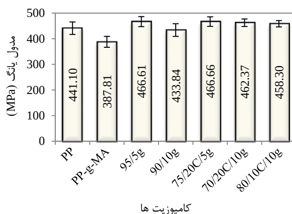
شکل ۱۰ مدول یانگ حالت‌های خالص و ترکیب‌های دوتایی و سه‌تایی پلی‌پروپیلن، PP-g-MA و \text{CaCO}_3
