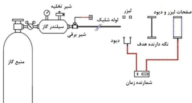
شکل ۴ طرح‌واره تفنگ گازی
