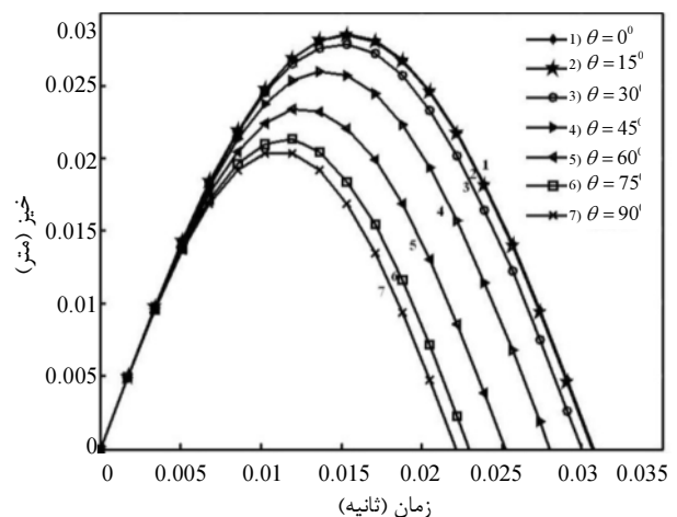
شکل ۱۶ تأثیر تغییر زاویه الیاف روی خیز ورق کامپوزیتی با لایه آلومینیوم (۱۰ و ۱) و جرم ضربه‌زننده بزرگ
