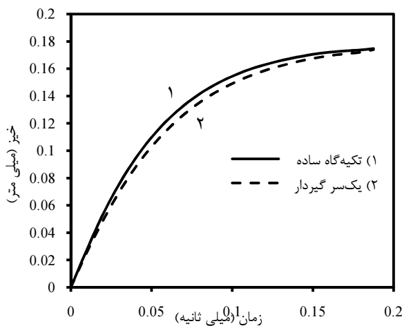
شکل ۸ مقایسه خیز ورق یکسرگیردار و تکیه گاه ساده
