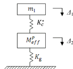
شکل ۲ مدل دو درجه آزادی جرم-فنر
