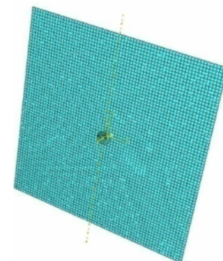
شکل ۵ مش بندی ورق و ضربه زننده
