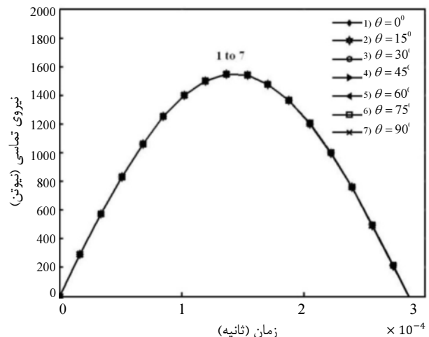
شکل ۱۵ تأثیر تغییر زاویه الیاف روی نیروی تماسی ورق کامپوزیتی با لایه آلومینیوم (۱۰ و ۱) و جرم ضربه‌زننده بزرگ
