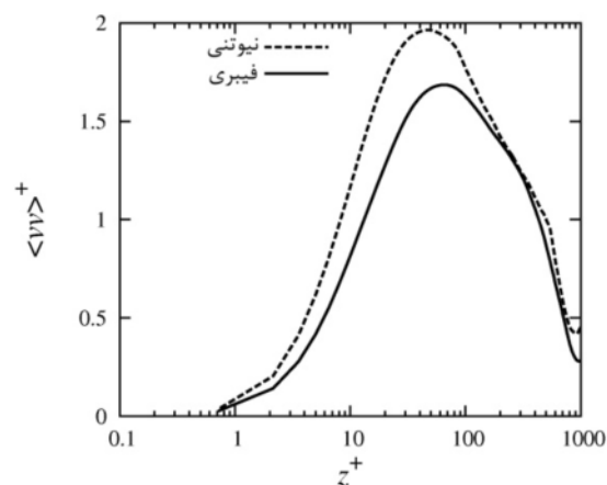
شکل ۶ تنش رینولدز در جهت عرضی به عنوان تابع فاصله از دیوار در مختصات درونی برای سیال نیوتنی و فیبری
