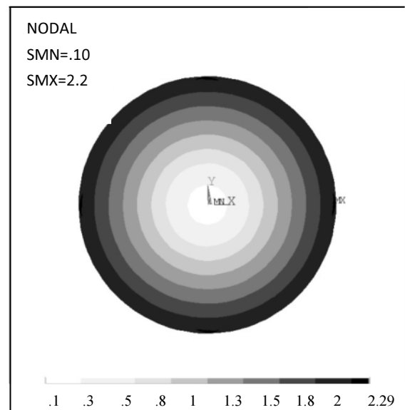
شکل ۷ نتیجه آنالیز عددی مغناطیسی میدان محیطی
