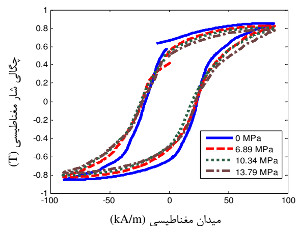
شکل ۳ نمودار چگالی شار مغناطیسی برحسب میدان مغناطیسی در پیش بارهای مکانیکی مختلف
