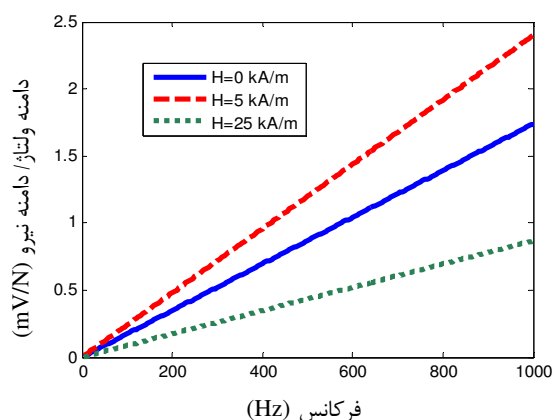
شکل ۱۲ نسبت دامنه ولتاژ حسگر به دامنه نیروی اعمالی (۱۰ N) در فرکانس‌های مختلف به‌ازای سه مقدار میدان مغناطیسی بایاس و بدون پیش‌تنش فشاری
