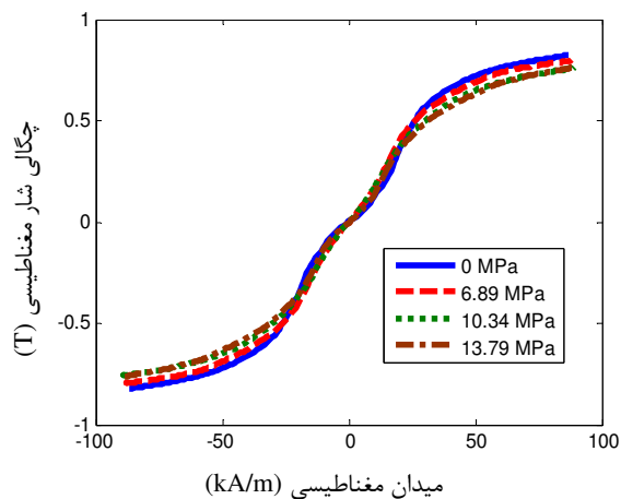
شکل ۵ نمودار بدون هیستریزیس چگالی شار مغناطیسی برحسب میدان مغناطیسی در پیش بارهای مکانیکی مختلف
