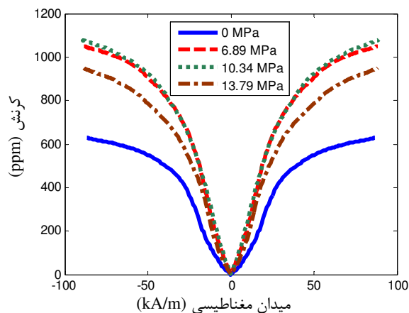
شکل ۶ نمودار بدون هیستریزیس کرنش محوری برحسب میدان مغناطیسی در پیش بارهای مکانیکی مختلف
