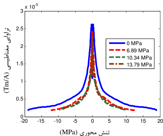
شکل ۱۰ نمودار تراوایی مغناطیسی ترفنل-دی نسبت برحسب تنش محوری در پیش بارهای مکانیکی مختلف
