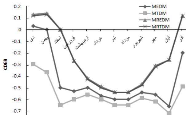
شکل ۱۳ کاهش انتشار آلودگی در ماه‌های سال در استراتژی مختلف، ساختمان ۵ طبقه
