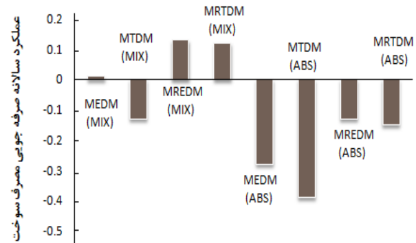
شکل ۲۰ عملکرد سالانه صرفه‌جویی مصرف سوخت در استراتژی مختلف (۵ طبقه)
