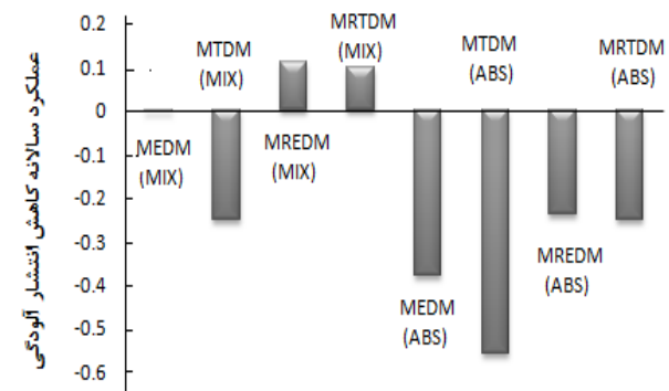
شکل ۲۱ میانگین سالانه کاهش انتشار آلودگی در استراتژی مختلف (۵ طبقه)
