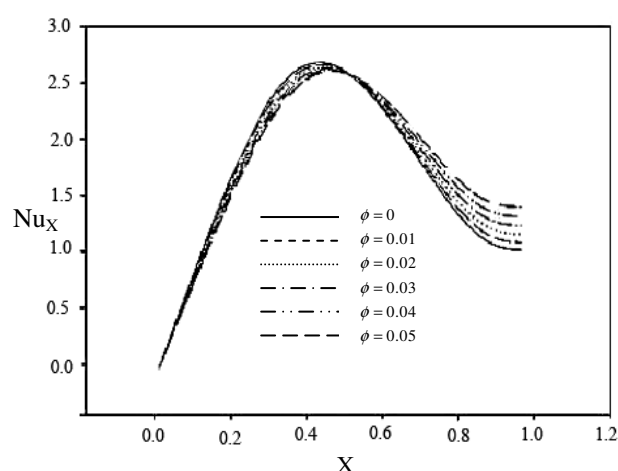
شکل ۷ تغییرات نوسلت موضعی به ازای درصد‌های حجمی مختلف نانوذرات ( \theta = 45^\circ , Ra = 10^4 , A = W/L = 0.5 )
