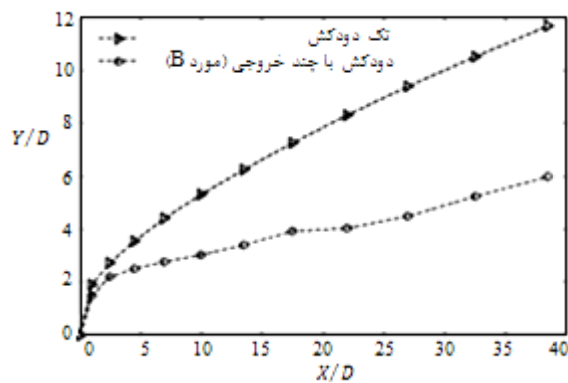
شکل ۱۰ نمایش خط مسیر دود خروجی از یک دودکش با یک چند خروجی
