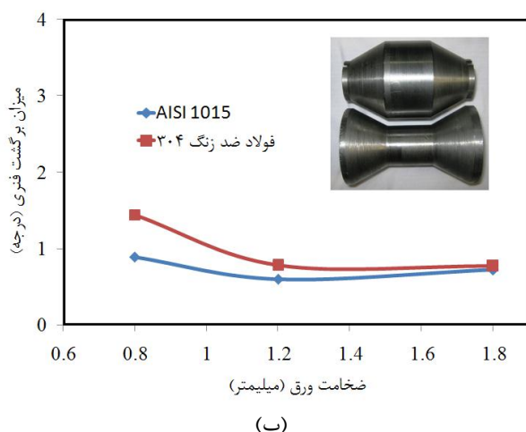
شکل ۹ مقادیر تجربی برگشت فنری برای دو هندسه غلتک بالایی الف- استوانه‌ای ب- دوزنقه‌ای
