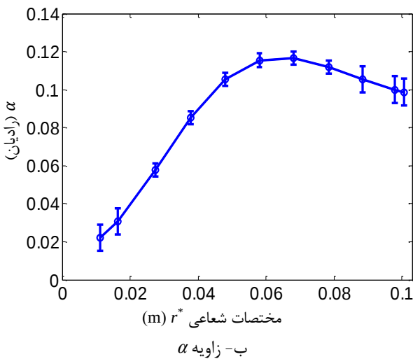
شکل پ- ۵ زاویه \alpha و مقدار سرعت شعاعی اندازه‌گیری شده بر روی خط جریان شماره ۳ و محدوده خطای آن
