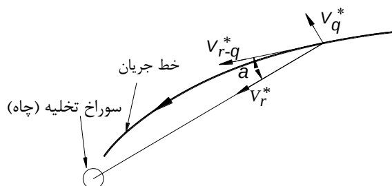
شکل ۲ زاویه بین بردار سرعت شعاعی و خط جریان ( \alpha ) و رابطه بین سرعت شعاعی و آزیموئال ( V_\theta^* = V_r^* \tan \alpha )
