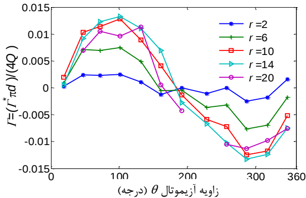
ج- تغییرات آزمونالی \Gamma در شعاعهای مختلف
