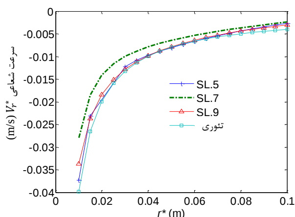
شکل پ-۴ سرعت شعاعی اندازه‌گیری شده بر روی خط جریان‌های ۵، ۷ و ۹ به همراه مقدار متوسط سرعت شعاعی از پیش‌بینی تئوری
