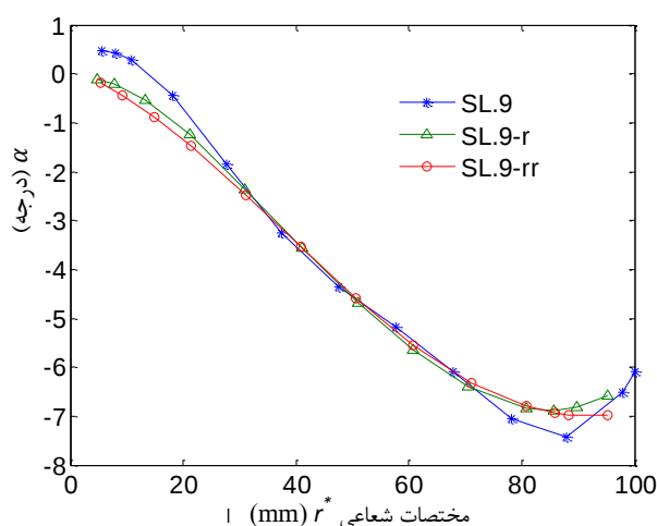
شکل پ-۲ زاویه \alpha مربوط خط جریان شماره ۹ با سه بار تکرار اندازه‌گیری با نرم‌افزار اتوکد
