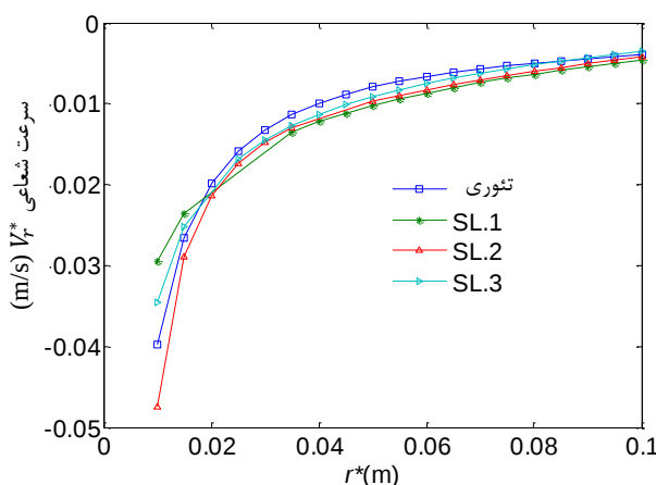
شکل پ-۳ سرعت شعاعی اندازه‌گیری شده بر روی خط جریان‌های شماره ۱، ۲ و ۳ به همراه مقدار متوسط سرعت شعاعی از پیش‌بینی تئوری
