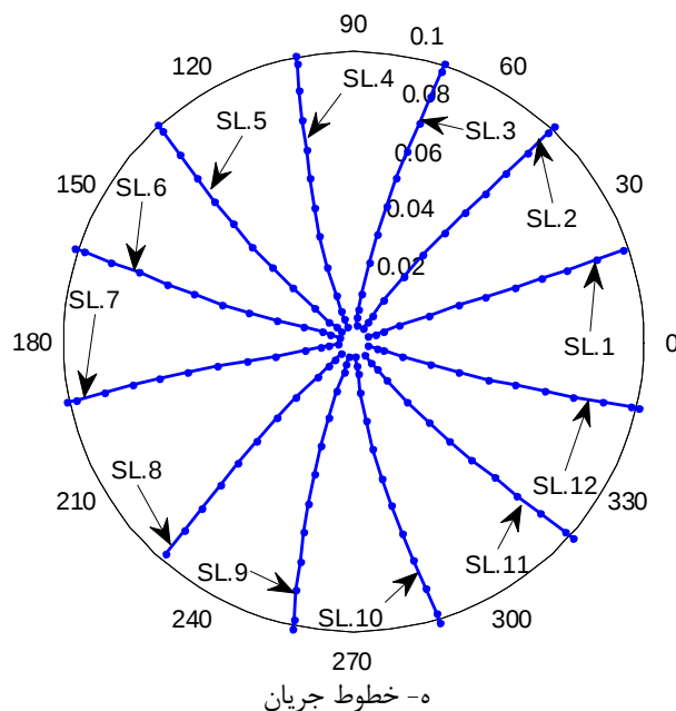
شکل ۸ الف تا د- تصاویر متوالی از نمای بالا و از حرکت توده رنگ در امتداد خطوط جریان ۱ تا ۱۲ در زمان‌های مختلف ه- خطوط جریان ۱ تا ۱۲ در صفحه r - \theta استخراج شده از نتایج آزمایش
