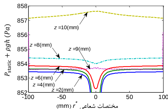
شکل ۷ تغییرات پارامتر P_{static} + \rho gh نسبت به فاصله از سوراخ خروجی ( r^* ) در ارتفاع‌های مختلف در صفحه \theta=90^\circ
