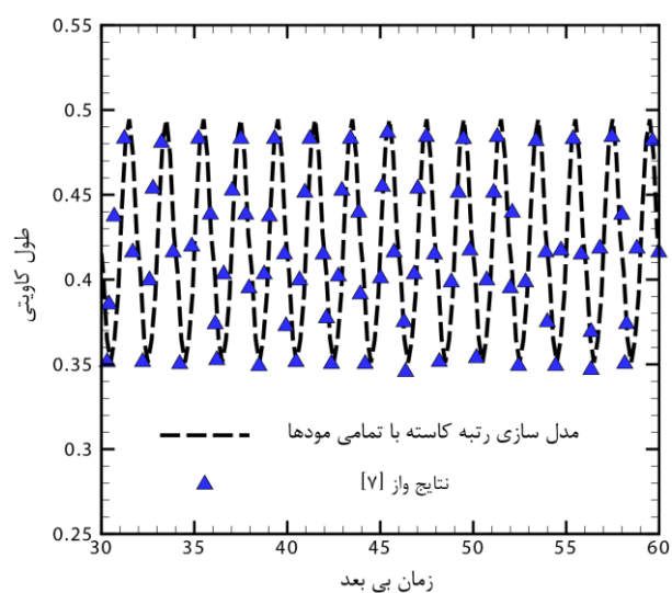
شکل ۸ تغییرات زمانی طول کاویتی ( \sigma = 1 و k = \pi/2 )
