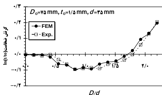
شکل ۷ نمودار تغییرات کرنش ضخامت برحسب فاصله از مرکز و مقایسه با نتایج آزمایشگاهی [۱۸، ۱۹]
