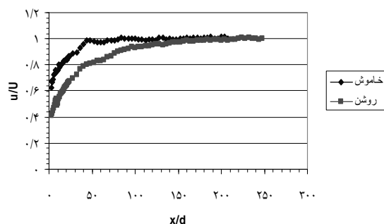
شکل ۶ توزیع سرعت بی بعد شده در جهت x پایین دست حسگر اول در حالت روشن و خاموش ( y/d=0 , U=5 m/s)
