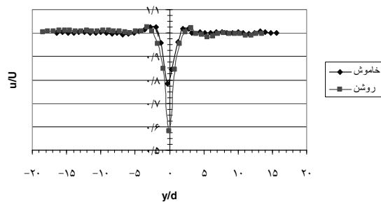
شکل ۵ توزیع بی بعد شده سرعت در جهت y پایین دست حسگر اول در حالت روشن و خاموش ( x/d=8 , U=10 m/s)
