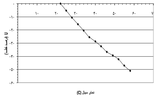
شکل ۸ تأثیر دمای محیط بر درصد خطای سرعت اندازه گیری شده ( U=10 m/s)
