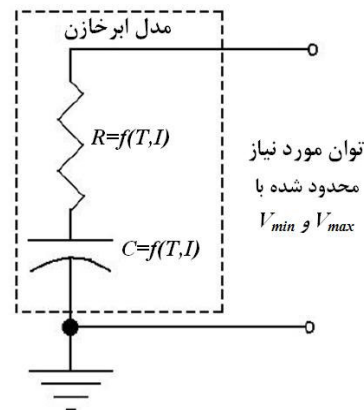
شکل ۱۱ مدل ابرخازن [۱۳]
