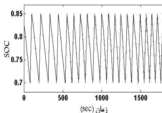
شکل ۱۹ تغییرات سطح شارژ ابرخازن‌ها در طول شبیه‌سازی
