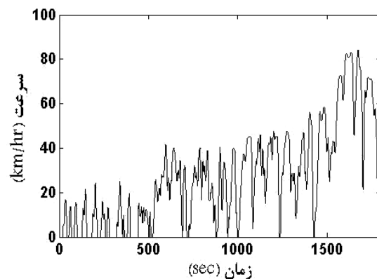
شکل ۸ سیکل رانندگی شهر تهران
