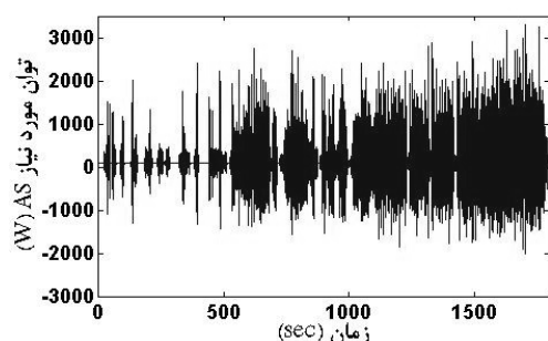
شکل ۱۵ توان مورد نیاز سیستم تعلیق فعال
