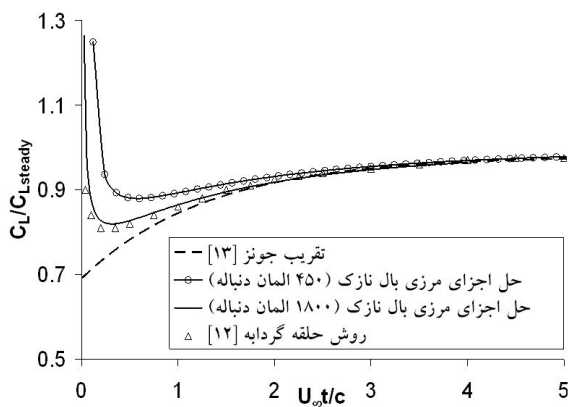
شکل ۲ تغییر ضریب برای گذرا برای بال تخت ( AR = 6 ) پس از شروع ناگهانی حرکت با سرعت ثابت
