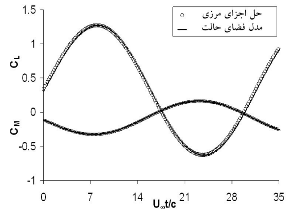
شکل ۸ تغییرات ضرایب برآ و ممان حول لبه حمله ایرفویل تخت در نوسان پیچشی حول مرکز ایرودینامیکی
