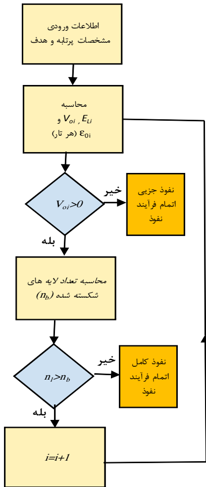
شکل ۴ روندنما محاسباتی تئوری ارائه‌شده
