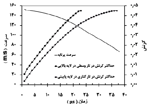
شکل ۶ تغییرات سرعت پرتابه، حداکثر کرنش در وسط تار در لایه بالایی و حداکثر کرنش در تار کناری در لایه پایینی ( V_i = 153 \text{ m/s} )
