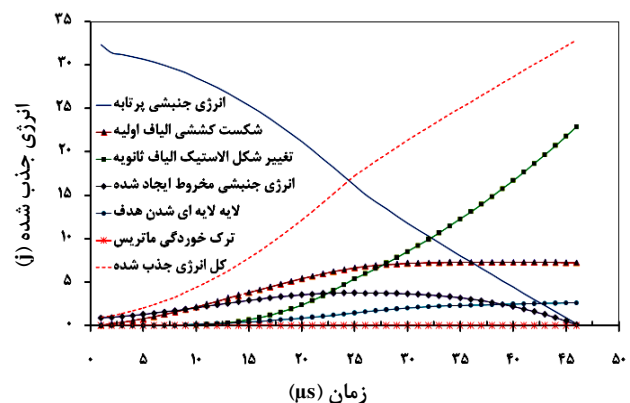
شکل ۷ انرژی جذب شده توسط مکانیزم‌های مختلف ( V_i = 152 \text{ m/s} )
