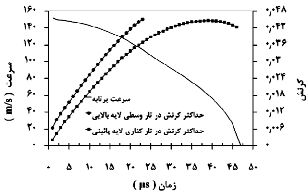
شکل ۸ تغییرات سرعت پرتابه، حداکثر کرنش در وسط تار در لایه بالایی و حداکثر کرنش در تار کناری در لایه پایینی
