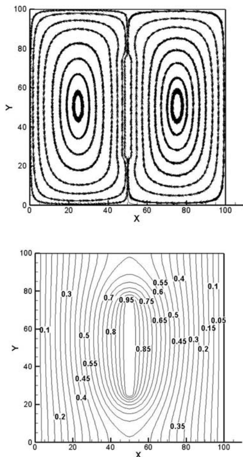
شکل ۶-۱ خطوط جریان و خطوط هم‌دما برای A_1=0.5 و A_2=0.5 ، گراش‌هف 10^3
