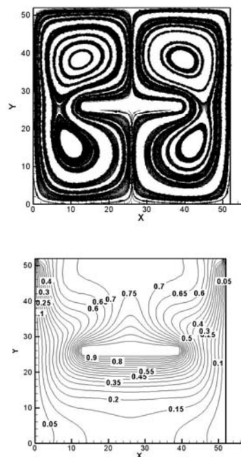
شکل ۵-۲ خطوط جریان و خطوط هم‌دما برای A_1=0.5 و A_2=0.5
