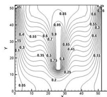
شکل ۶-۳ خطوط جریان و خطوط هم‌دما برای A=0/5 و A_1=0/5
