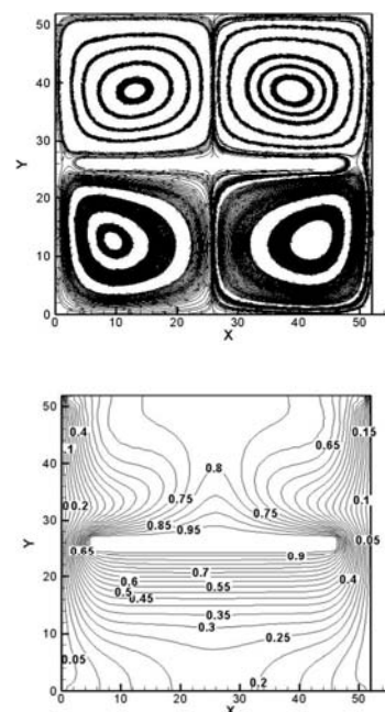
شکل ۵-۳ خطوط جریان و خطوط هم‌دما برای A_1=0.5 و A_2=0.8
