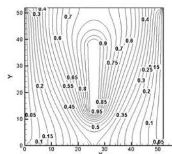
شکل ۶-۲ خطوط جریان و خطوط هم‌دما برای A=0/5
