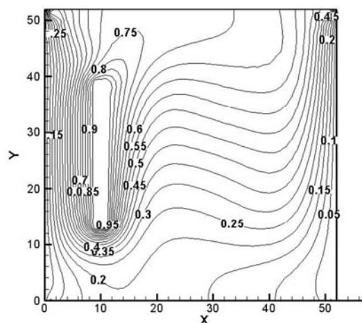
شکل ۷-۱ خطوط جریان و خطوط هم‌دما برای عدد گراش‌هف 10^5 .
