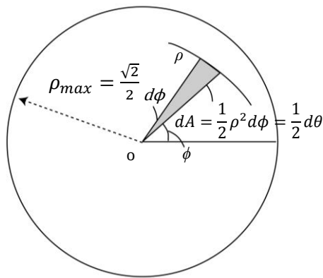
شکل ۳ مختصات قطبی ρ-φ
