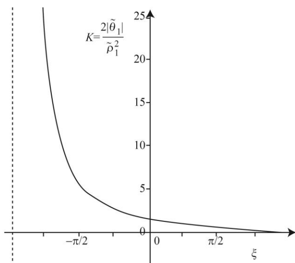
شکل ۷ تغییرات K = \frac{2|\tilde{\theta}_1|}{\tilde{\rho}_1^2} بر حسب \xi
