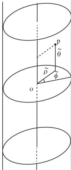
شکل ۶ مختصات استوانه‌ای (\tilde{\rho}, \tilde{\phi}, \tilde{\theta})
