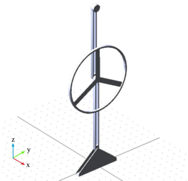
شکل ۴ مدل شبیه‌سازی شده از پاندول معکوس دوگانه با چرخ عکس‌عملی در نرم‌افزار آدامز
