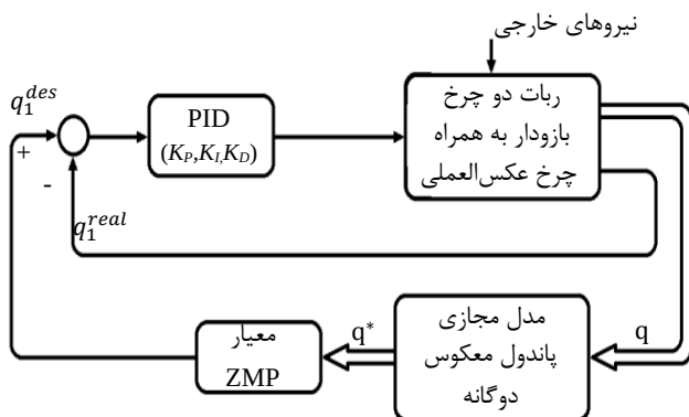
شکل ۱۳ بلوک دیاگرام کنترلی بخش پایدارساز
