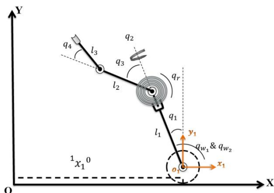
شکل ۲ طرح کلی ربات دو چرخ بازودار به همراه چرخ عکس‌العملی
