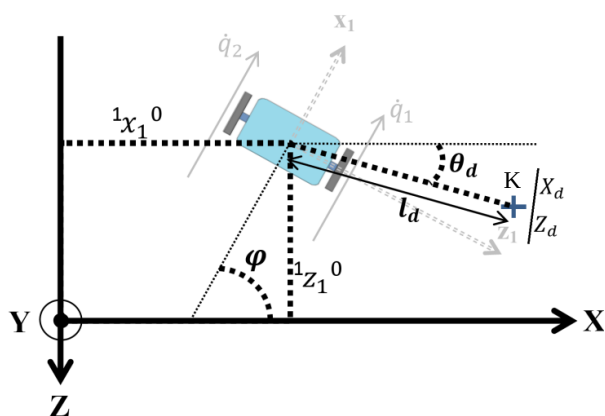
شکل ۱۴ پایه متحرک ربات و پارامترهای مورد نیاز جهت کنترل مسیر حرکت زمانی
