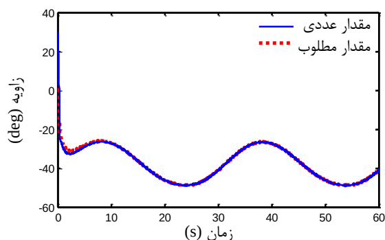
شکل ۱۷ منحنی تغییرات زاویه بدنه اصلی ربات و نقطه مطلوب آن
