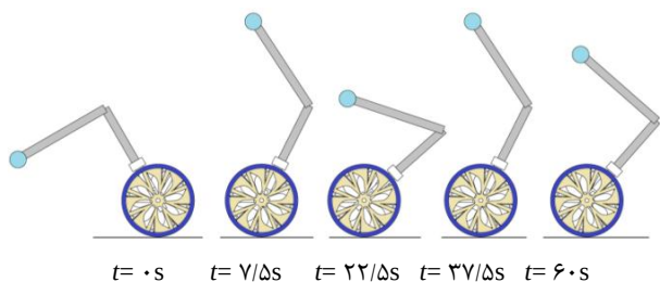
شکل ۱۹ تصویر ربات در طول زمان و اصلاح حالت خود حین پایدارسازی
