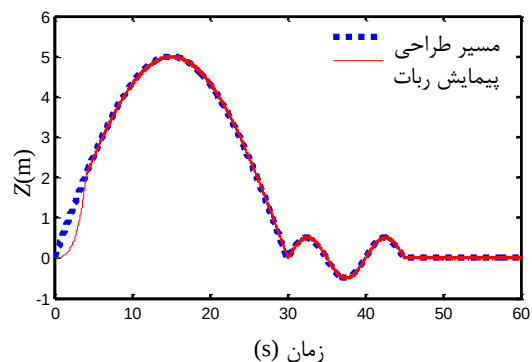
شکل ۲۸ منحنی پارامتر Z در طول زمان و نحوه تعقیب ربات بر روی آن
