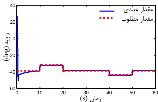
شکل ۲۱ منحنی تغییرات زاویه بدنه اصلی ربات و اصلاح نقطه مطلوب آن برای رسیدن حالت سیستم از شرایط موجود به حالت پایدار طبیعی طبق معیار نقطه صفر گشتاوری
