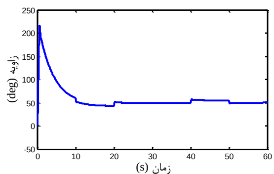
شکل ۲۲ منحنی تغییرات دورانی چرخ عکس‌عملی حین پایداری و اصلاح حالت ربات
