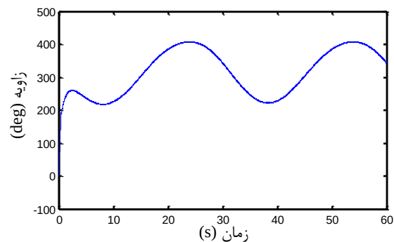
شکل ۱۸ منحنی تغییرات دورانی چرخ عکس‌العملی
