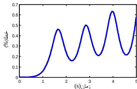
شکل ۱۰ خطای حاصل از نتایج تحلیلی و عددی برای میزان تغییرات زاویه بدنه اصلی ربات
