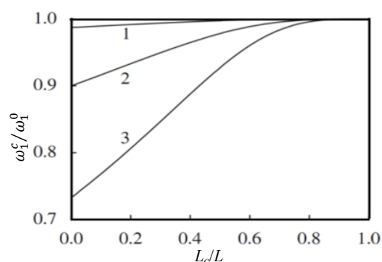
الف- نسبت فرکانس طبیعی اول تیر ترک‌دار به بدون ترک
