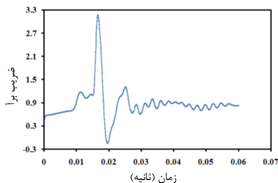
شکل ۲۴ ضریب برآ روی پره در زاویه ۳۰ درجه با روش SA
