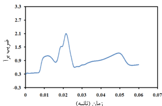
شکل ۲۲ ضریب برآ روی پره در زاویه ۲۰ درجه با روش SA
