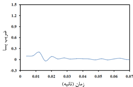
شکل ۱۹ ضریب پسا روی پره در زاویه ۴۵ درجه با روش DDES
