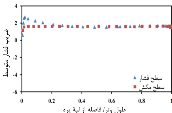
شکل ۱۱ توزیع ضریب فشار روی پره در زاویه ۴۵ درجه با روش DDES
