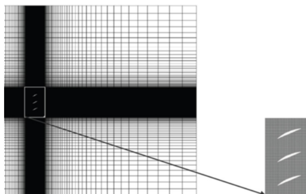
شکل ۲ شبکه‌بندی میدان حل جریان سیال
