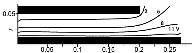
شکل ۷ توزیع پتانسیل الکتریکی در پلاسما
