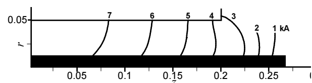
شکل ۵ توزیع جریان الکتریکی محصور بین دو الکترودها
