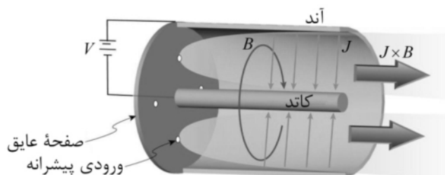
شکل ۱ طرح‌واره‌ای از یک رانشگر MPD [۲]
