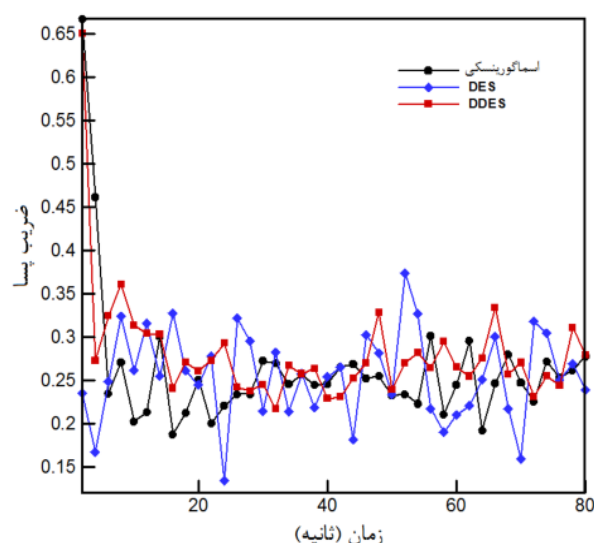
شکل ۲۳ ضریب پسای ساختمانی با ابعاد واحد در رینولدز ۲۲۰۰۰ با استفاده از مدل‌های مختلف توربولانسی
