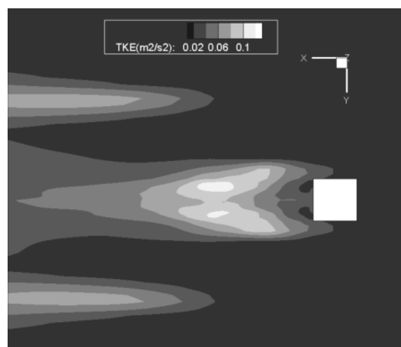
شکل ۲۰ مقدار انرژی توربولانسی در صفحه z = 0.5 با استفاده از مدل اسمآگورینسکی
