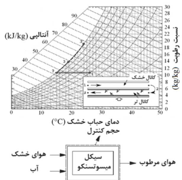
شکل 2 نمودار سایکرومتریک به همراه اصول کار مبدل و حجم کنترل بر اساس چرخه میسوتسنکو [14, 15]
