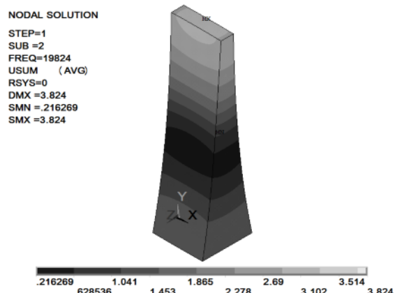
شکل ۱۵ فرکانس طبیعی ارتعاشات طولی و نسبت جابه‌جایی نواحی مختلف برای متمرکزکننده اصلاح نشده
