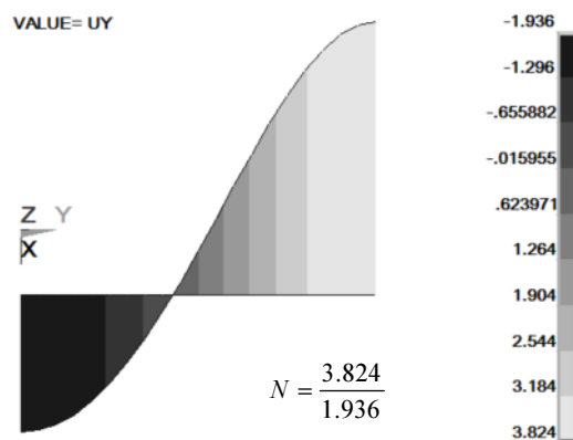
شکل ۱۶ جابه‌جایی نسبی متمرکزکننده در راستای طول آن برای متمرکزکننده اصلاح نشده
