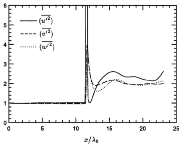
شکل ۱۰ تغییرات شدت اغتشاشات در عبور از موج ضربه‌ای با ماخ
