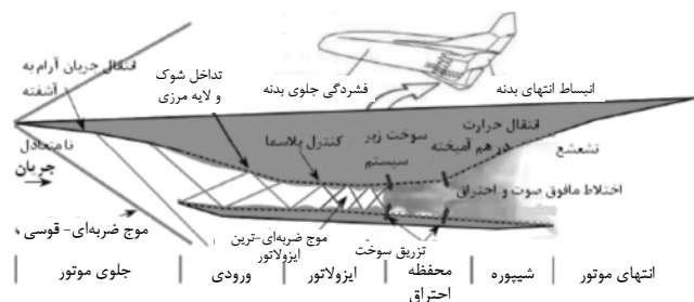
شکل ۱ موتور اسکرم جت [۱]
