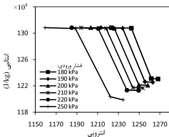
شکل ۲۰ تغییرات انتالی بر حسب انتروپی
